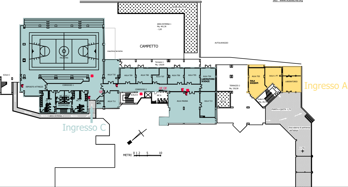
PIANTA PIANO TERRA a quota -1,75
